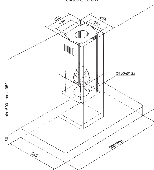
Okap ATOLL
