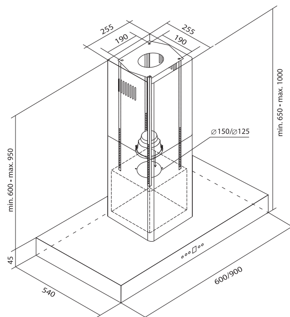
Okap CEJLON
