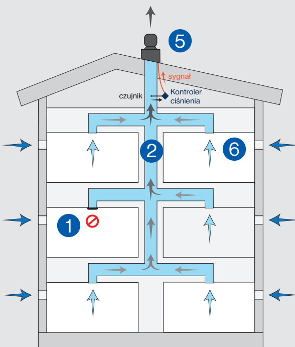
Przykład budynku z Kontrolerem ciśnienia VILPE 24 V
