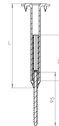
VILPE® łącznik Croco A + regulowana śruba 95. L to długość łącznika Croco.
