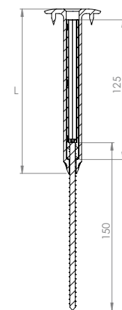
VILPE® łącznik Croco A + regulowana śruba 150. L to długość łącznika Croco.
