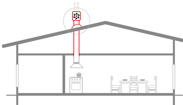
Okap kuchenny z wentylatorem na dachu – CICHAKUCHNIA VILPE®
